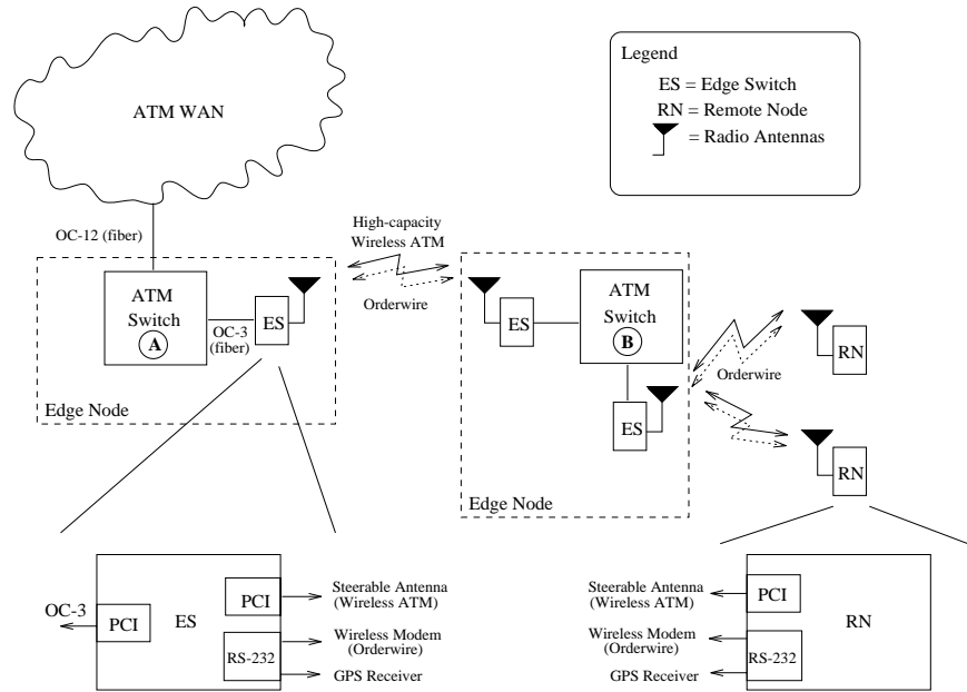
Figure 3: Edge Nodes and Edge Switches.
